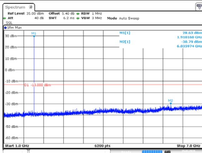
GSM1900_810
