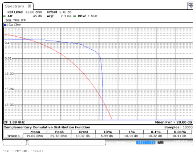
EGPRS1900_810
