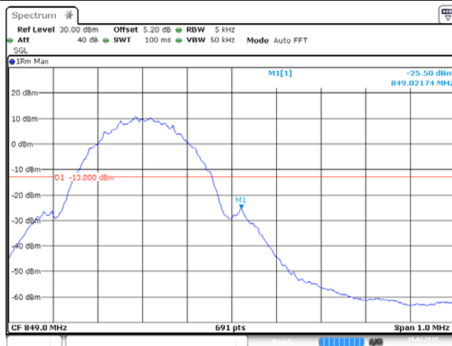
GSM850_251
