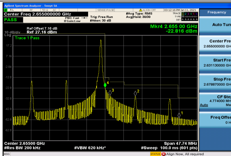
Band41-20MHz-QPSK-41140-1RB#99
