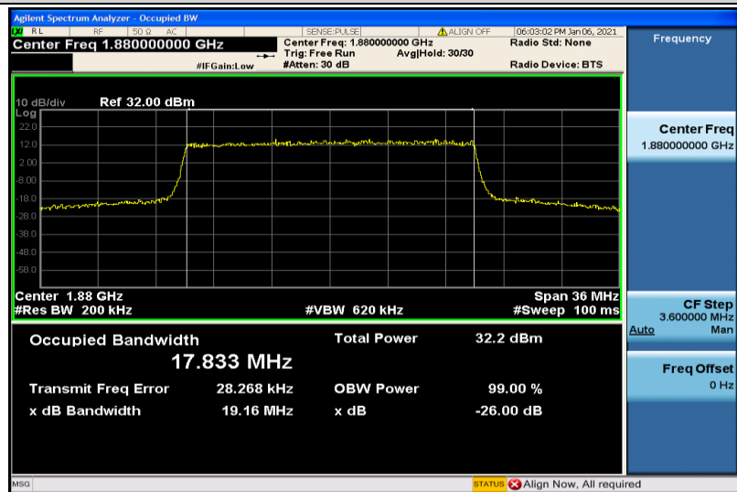
Band2-20MHz-QPSK-18900-100RB#0-17.833
