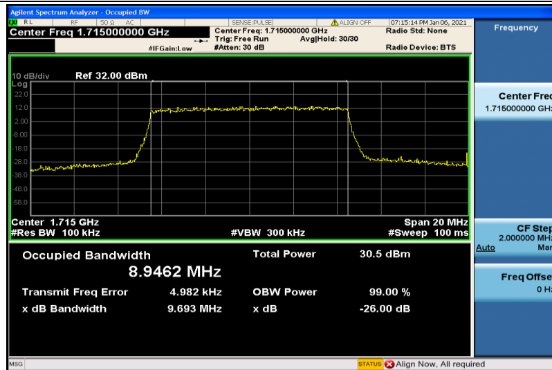
Band4-10MHz-QPSK-20000-50RB#0-8.9462
