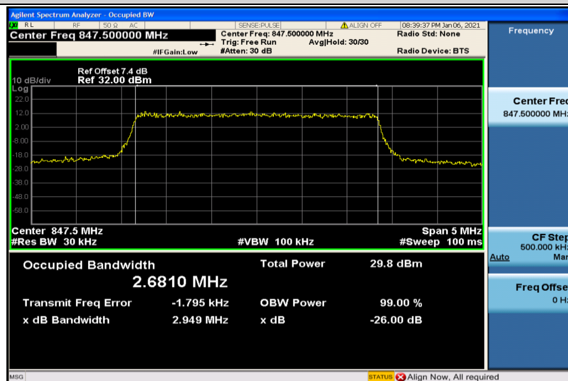
Band5-3MHz-QPSK-20635-15RB#0-2.6810
