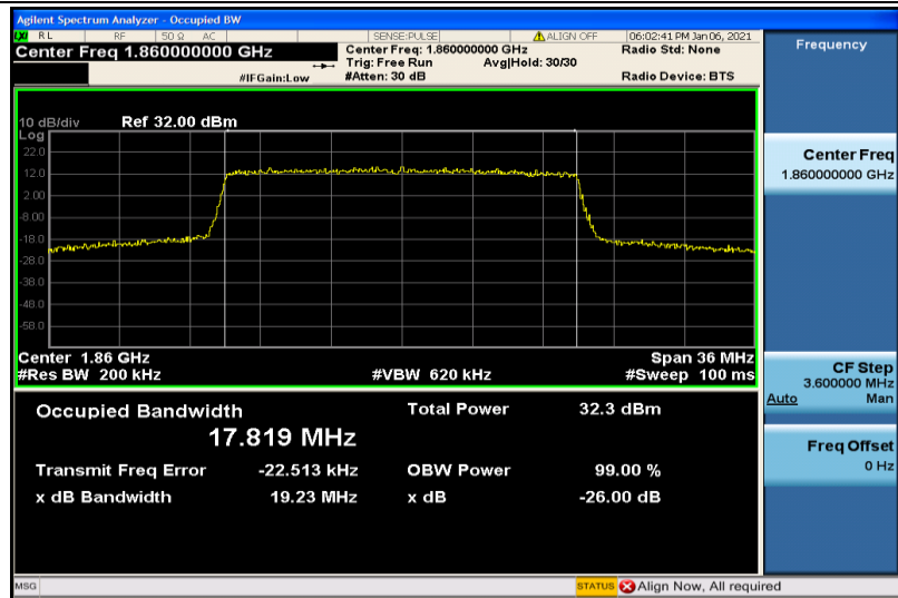
Band2-20MHz-QPSK-18700-100RB#0-17.819
