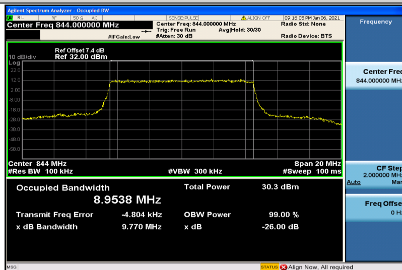
Band5-10MHz-QPSK-20600-50RB#0-8.9538
