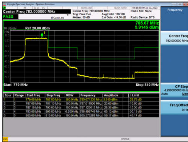
FDD13-10MHz-QPSK-MCH-1RB#0
