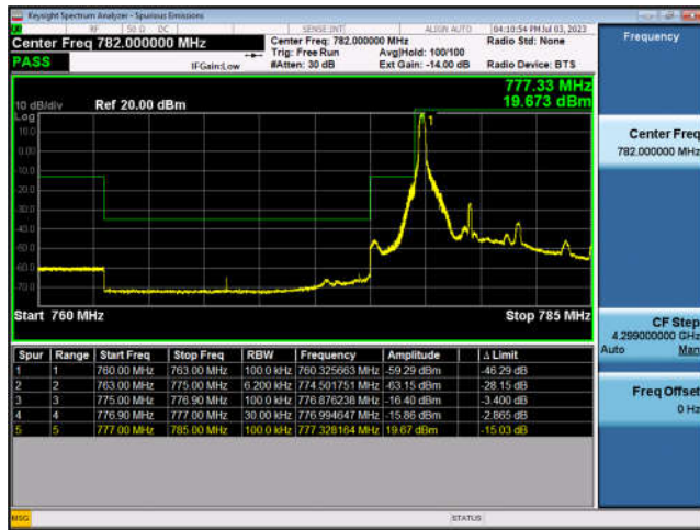
FDD13-5MHz-QPSK-LCH-25RB#0
