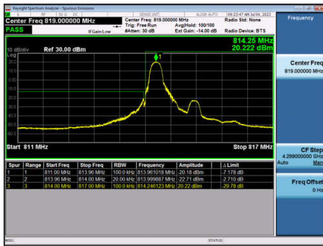
FDD26-Part 90-1.4MHz-QPSK-LCH-6RB#0
