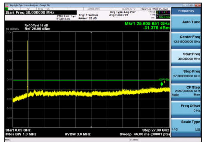
TDD41_HighRange_20MHz_30MHz~27GHz
