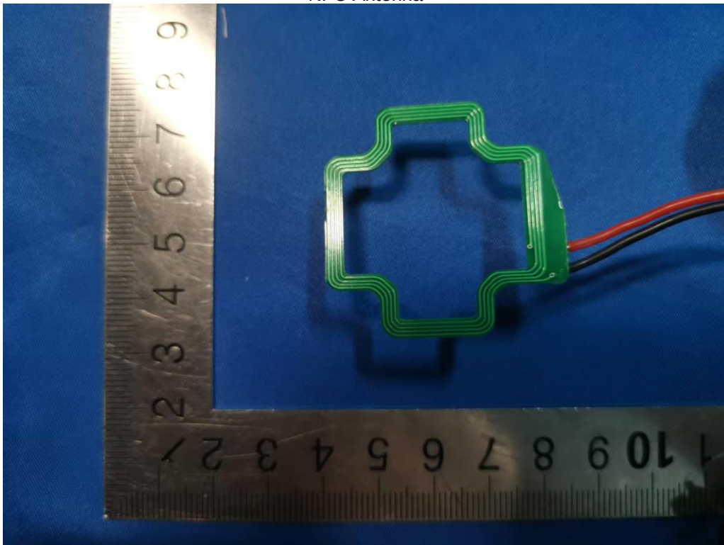
NFC Antenna
