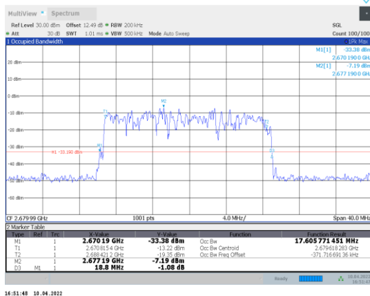
1-N41-PC3-30-20-H-5-CP-QPSK-Outet_Full-51@0-A nt1-17.606-18.800-≤20-PASS
