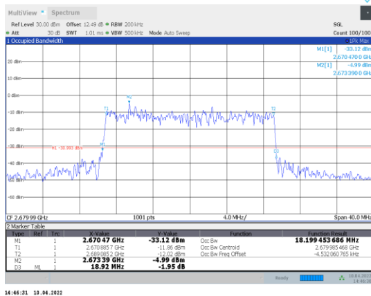
1-N41-PC3-30-20-H-3-DFT-16QAM-Outet_Full-50@0-A nt1-18.199-18.920-≤20-PASS
