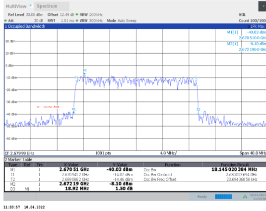
1-N41-PC3-30-20-H-1-DFT-QPSK-Outet_Full-50@0-A nt1-18.145-18.920-≤20-PASS
