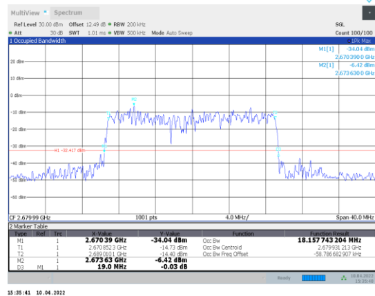
1-N41-PC3-30-20-H-4-DFT-64QAM-Outet_Full-50@0-A nt1-18.158-19.000-≤20-PASS
