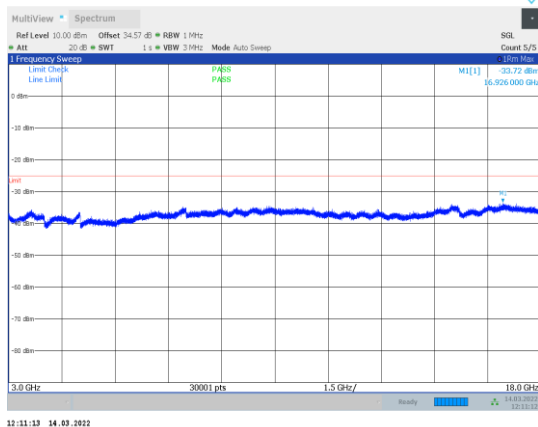
1-N41-PC3-30-100-L-2-CP-OFDM QPSK-Edge_1RB_Right-1 @272-3000-18000-Ant1--33.72--25-PASS
