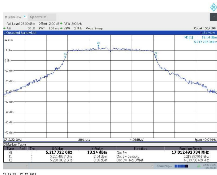
11a Ant11 5220
