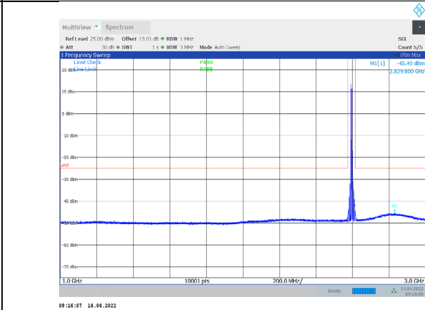
1-N38-PC3-30-10-M-1-CP-QPSK-Edge_1RB_Left-1@0 1000-3000-Ant1--45.49--25-PASS
