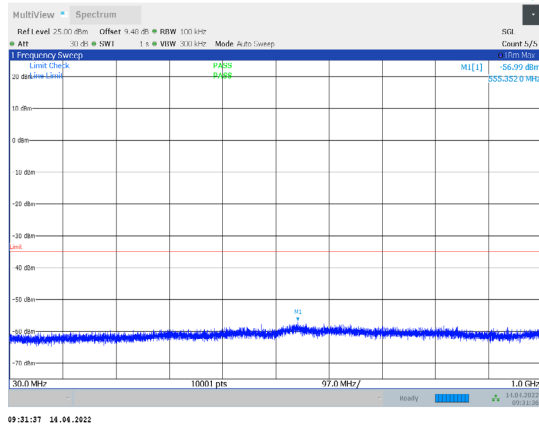
1-N38-PC3-30-15-L-3-CP-QPSK-Outer_Full-38@0-30- 1000-Ant1--56.99--35-PASS
