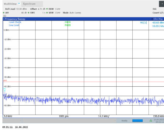
1-N38-PC3-30-15-L-3-CP-QPSK-Outer_Full-38@0-0.0 09-0.15-Ant1--65.65--55-PASS
