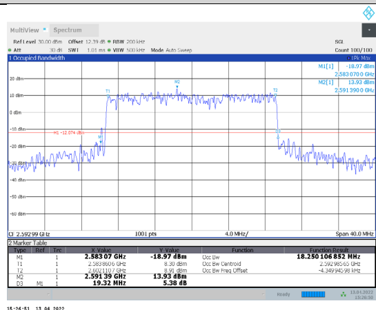
1-N41-PC3-30-20-M-3-CP-64QAM-Outer_Full-51@0-A nt1-18.25-19.320-≤20-PASS
