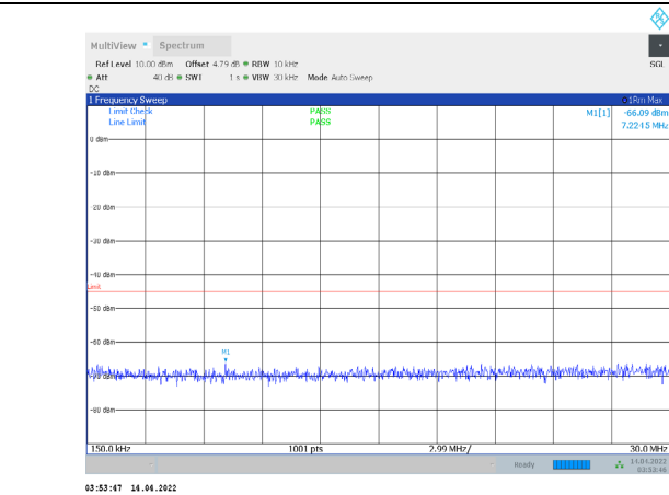
1-N41-PC3-30-20-L-2-CP-QPSK-Edge_1RB_Right-1@5 0-0.15-30-Ant1--66.09--45-PASS
