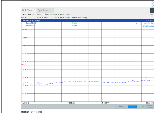
1-N41-PC3-30-20-L-2-CP-QPSK-Edge_1RB_Right-1@ 50-3000-18000-Ant1--42.99--25-PASS
