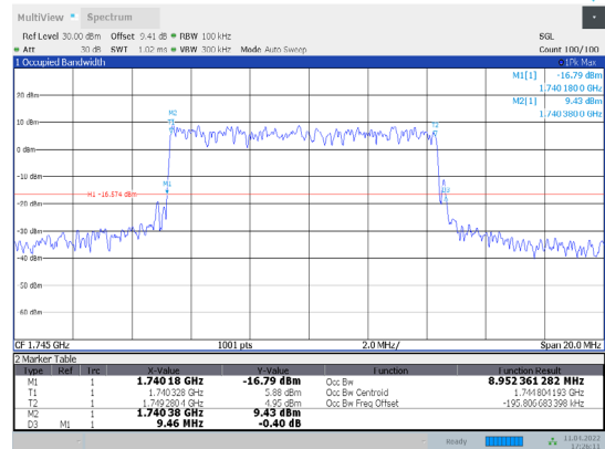
1-N66-PC3-15-10-M-1-CP-QPSK-Outer_Full-50@0-A 1-8.952-9.460-≤10-PASS
