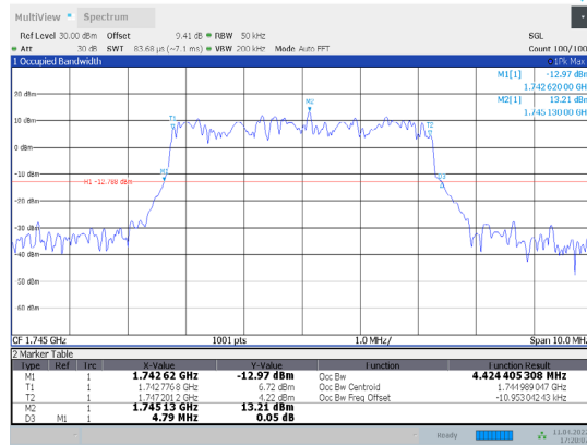
1-N66-PC3-15-5-M-6-DFT-QPSK-Out_ Full-25@0-A nt1-4.424-4.790-≤5-PASS
