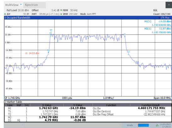
1-N66-PC3-15-5-M-7-DFT-16QAM-Out_ Full-25@0-A nt1-4.46-4.790-≤5-PASS
