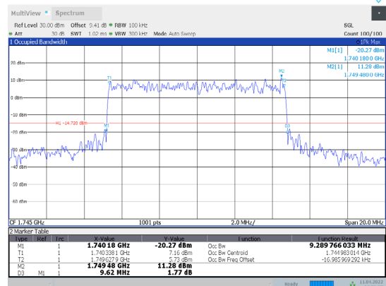
1-N66-PC3-15-10-M-3-CP-64QAM-Outer_Full-52@0-A nt1-9.29-9.620-≤10-PASS
