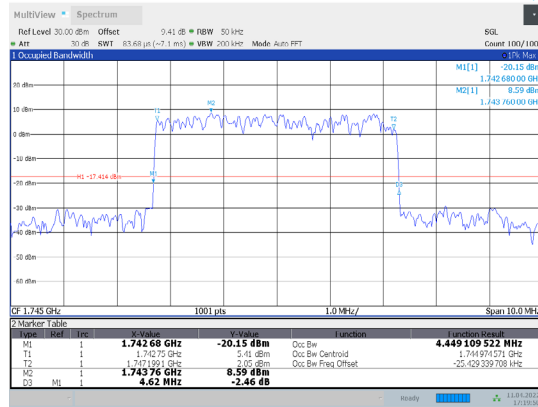
1-N66-PC3-15-5-M-4-CP-256QAM-Out_ Full-25@0-A nt1-4.449-4.620-≤5-PASS
