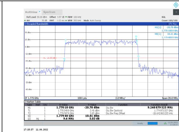
1-N66-PC3-15-10-H-2-CP-16QAM-Outer_Full-52@0-Ant1 -9.249-9.600≤10-PASS
