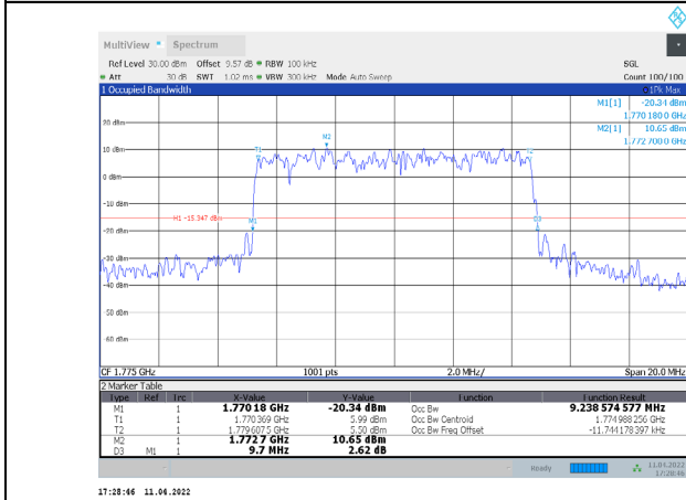
1-N66-PC3-15-10-H-3-CP-64QAM-Outer_Full-52@0-Ant1 1-9.239-9.700≤10-PASS
