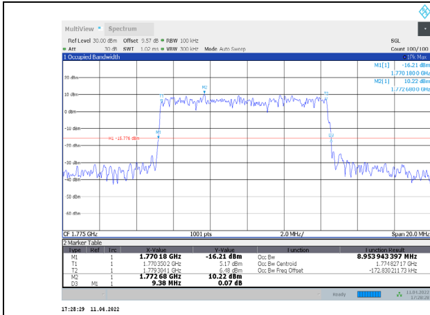
1-N66-PC3-15-10-H-1-CP-QPSK-Outer_Full-50@0-Ant1 -8.954-9.380≤10-PASS
