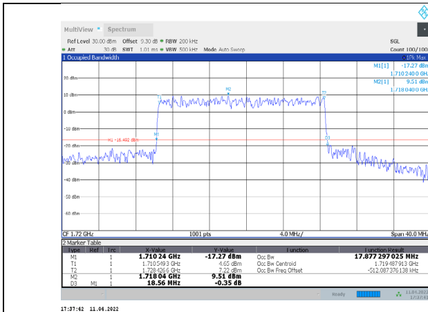
1-N66-PC3-15-20-L-1-CP-QPSK-Outer_Full-100@0-Ant 1-17.877-18.560-≤20-PASS
