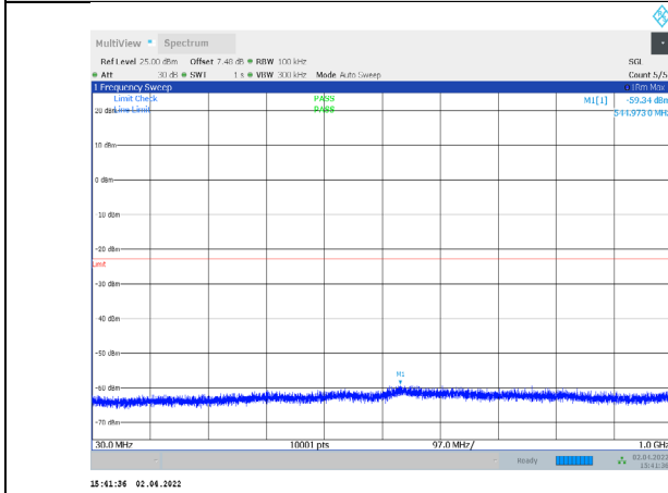
1-N66-PC3-15-5-L-3-CP-QPSK-Outer_Full-25@0-30-1 000-Ant1--59.34--23-PASS
