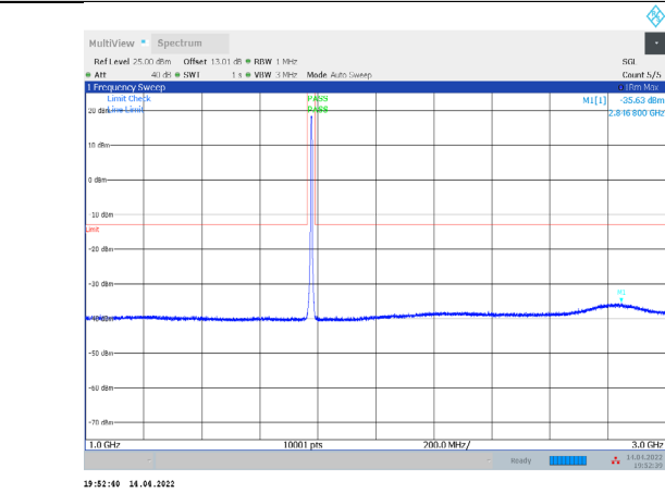
1-N66-PC3-15-5-H-3-CP-QPSK-Outter_Full-25@0-1000- 3000-Ant1--35.63--13-PASS
