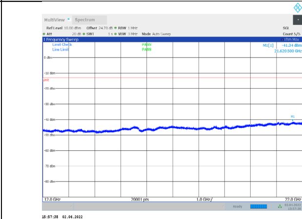
1-N66-PC3-15-15-M-1-CP-QPSK-Edge_1RB_Left-1@0- 12000-22000-Ant1--41.34--13-PASS
