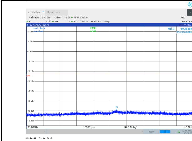
1-N66-PC3-15-5-H-3-CP-QPSK-Outter_Full-25@0-30-1 000-Ant1--59.36--23-PASS
