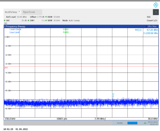
1-N66-PC3-15-15-H-1-CP-QPSK-Edge_1RB_Left-1@0- 0.15-30-Ant1--67.30--33-PASS
