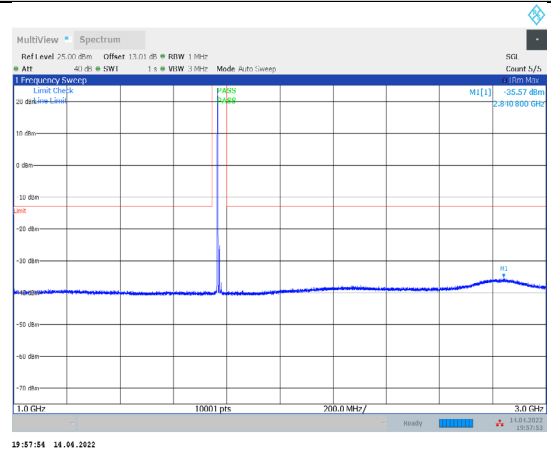
1-N66-PC3-15-15-H-1-CP-QPSK-Edge_1RB_Left-1@0- 1000-3000-Ant1--35.57--13-PASS
