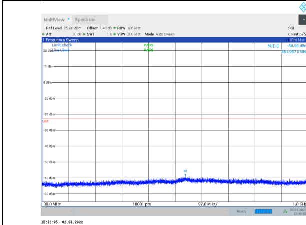
1-N66-PC3-15-5-M-3-CP-QPSK-Outer_Full-25@0-30-1 000-Ant1--58.96--23-PASS
