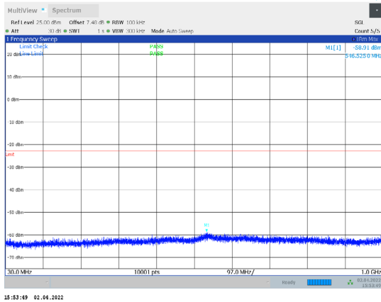
1-N66-PC3-15-15-L-2-CP-QPSK-Edge_1RB_Right-1@ 78-30-1000-Ant1--58.91--23-PASS
