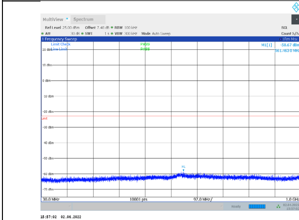
1-N66-PC3-15-15-M-1-CP-QPSK-Edge_1RB_Left-1@0 -30-1000-Ant1--58.67--23-PASS
