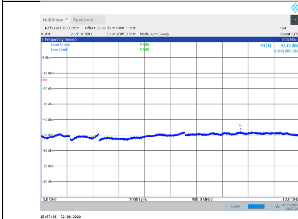
1-N66-PC3-15-15-M-1-CP-QPSK-Edge_1RB_Left-1@0 -3000-12000-Ant1--47.18--13-PASS
