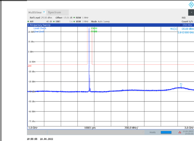
1-N66-PC3-15-15-M-1-CP-QPSK-Edge_1RB_Left-1@0- 1000-3000-Ant1--35.68--13-PASS
