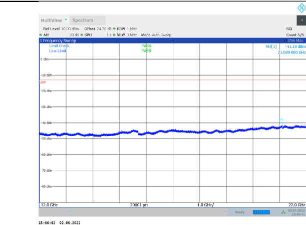
1-N66-PC3-15-5-M-3-CP-QPSK-Outer_Full-25@0-1200 0-22000-Ant1--41.18--13-PASS
