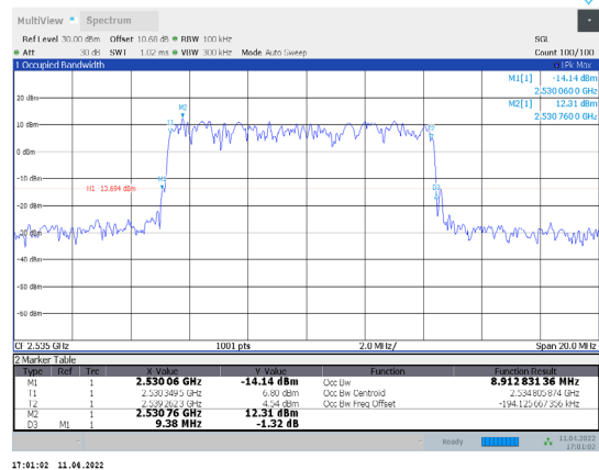
1-N7-PC3-15-10-M-9-DFT-256QAM-Outet_Full-50@0-A nt1-8.913-9.380-≤10-PASS
