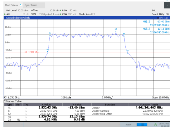
1-N7-PC3-15-5-M-5-DFT-PI/2BPSK-Outer_Full-25@0-A nt1-4.461-4.820-≤5-PASS
