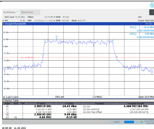
1-N7-PC3-15-5-H-3-CP-64QAM-Outer_Full-25@0-Ant1- 4.467-4.840-≤5-PASS
