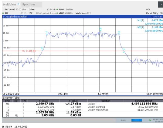
1-N7-PC3-15-5-L-7-DFT-16QAM-Outer_Full-25@0-Ant1 -4.497-5.050-≤5-PASS
