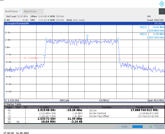
1-N7-PC3-15-20-M-1-CP-QPSK-Outer_Full-100@0-A nt1-17.889-18.640-≤20-PASS
