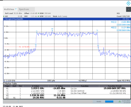
1-N7-PC3-15-20-M-3-CP-64QAM-Outer_Full-106@0-A nt1-19-19.560-≤20-PASS
