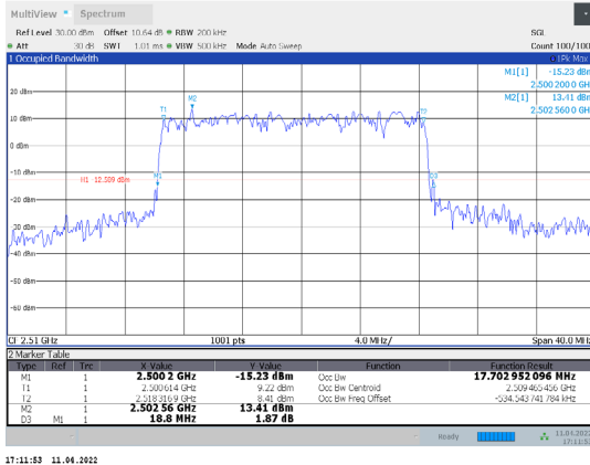
1-N7-PC3-15-20-L-7-DFT-16QAM-Outer_Full-100@0-A nt1-17.703-18.800-≤20-PASS
