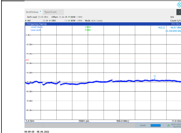
1-N7-PC3-15-5-L-2-CP-QPSK-Edge_1RB_Right-1@24 -3000-12000-Ant1--46.87--25-PASS
