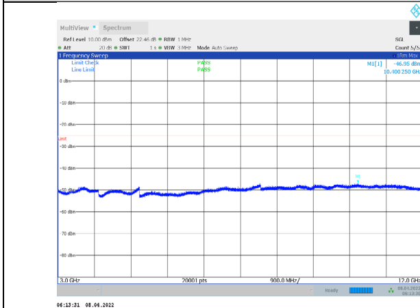
1-N7-PC3-15-5-M-2-CP-QPSK-Edge_1RB_Right-1@24 -3000-12000-Ant1--46.95--25-PASS
