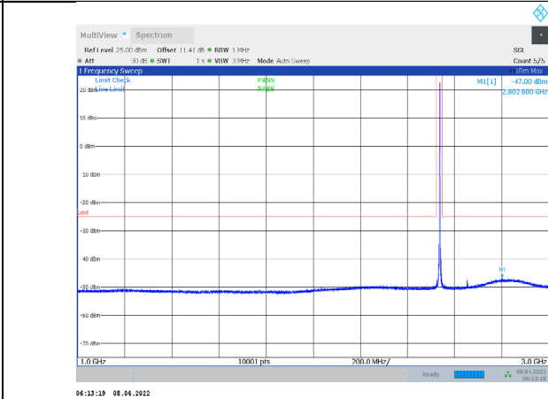
1-N7-PC3-15-5-M-2-CP-QPSK-Edge_1RB_Right-1@24 1000-3000-Ant1--47.00--25-PASS
