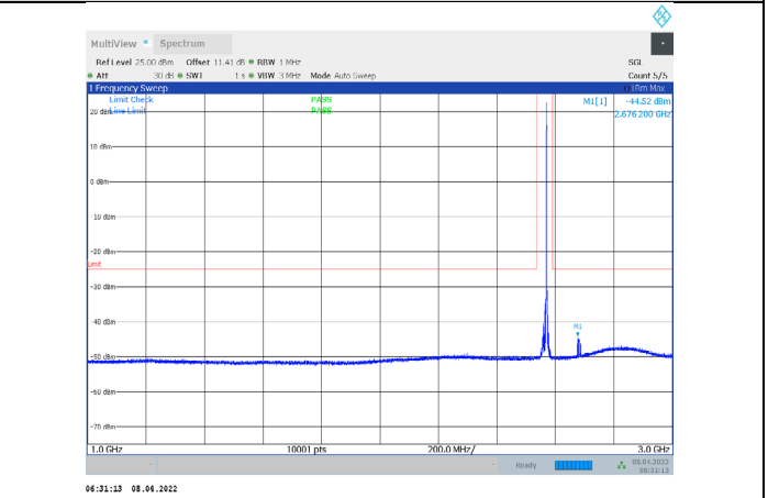
1-N7-PC3-15-15-H-2-CP-QPSK-Edge_1RB_Right-1@7 8-1000-3000-Ant1--44.52--25-PASS
