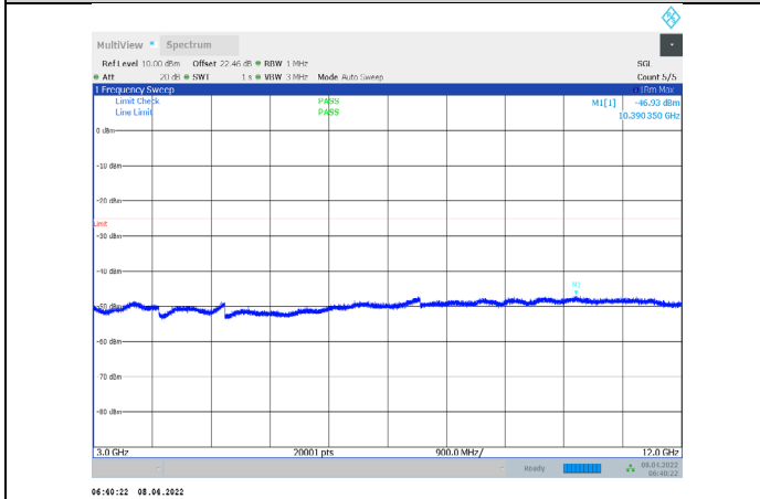
1-N7-PC3-15-20-M-2-CP-QPSK-Edge_1RB_Right-1@1 05-3000-12000-Ant1--46.93--25-PASS
