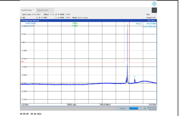
1-N7-PC3-15-20-H-2-CP-QPSK-Edge_1RB_Right-1@1 05-1000-3000-Ant1--44.70--25-PASS
