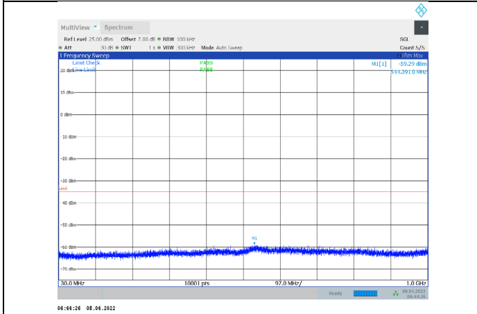
1-N7-PC3-15-20-H-2-CP-QPSK-Edge_1RB_Right-1@1 05-30-1000-Ant1--59.29--35-PASS
