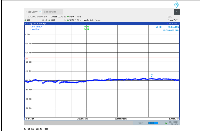
1-N7-PC3-15-20-H-2-CP-QPSK-Edge_1RB_Right-1@1 05-3000-12000-Ant1--46.85--25-PASS
