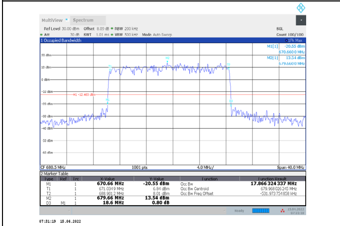
1-N71-PC3-15-20-M-6-DFT-QPSK-Outer_Full-100@0-Ant1-17.866-18.600-≤20-PASS
