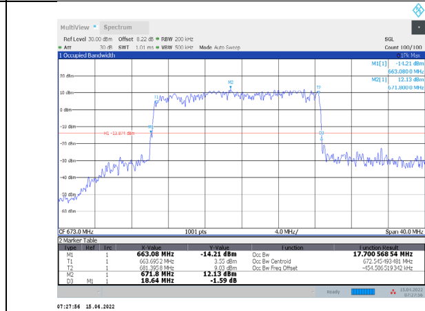
1-N71-PC3-15-20-L-6-DFT-QPSK-Outer_Full-100@0-Ant1 1-17.701-18.640-≤20-PASS
