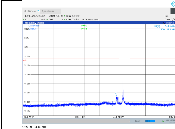
1-N71-PC3-15-20-L-1-CP-QPSK-Edge_1RB_Left-1@0 -30-1000-Ant1--54.24--13-PASS
