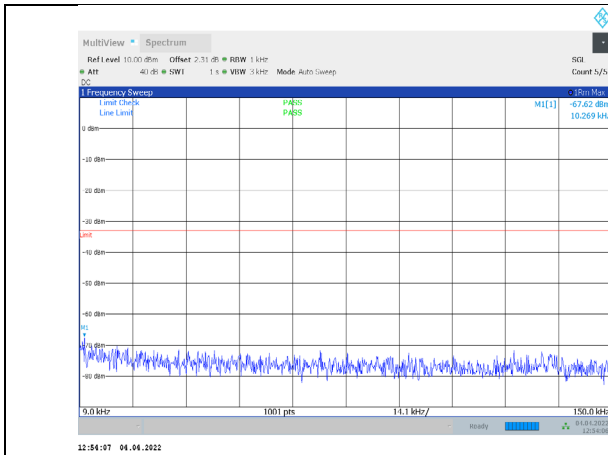
1-N71-PC3-15-20-L-1-CP-QPSK-Edge_1RB_Left-1@0 -0.009-0.15-Ant1--67.62--33-PASS
