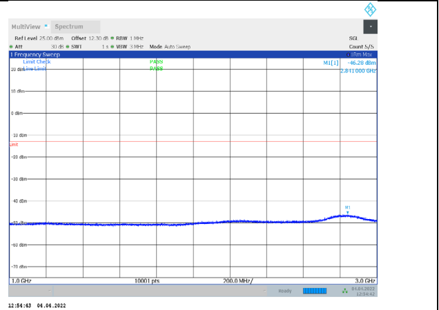
1-N71-PC3-15-20-L-1-CP-QPSK-Edge_1RB_Left-1@0-1 000-3000-Ant1--46.28--13-PASS
