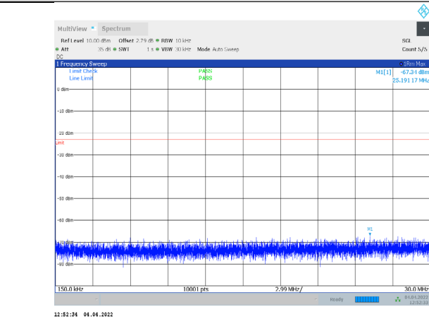
1-N71-PC3-15-15-H-3-CP-QPSK-Outer_Full-79@0.0.15 -30-Ant1--67.34--23-PASS
