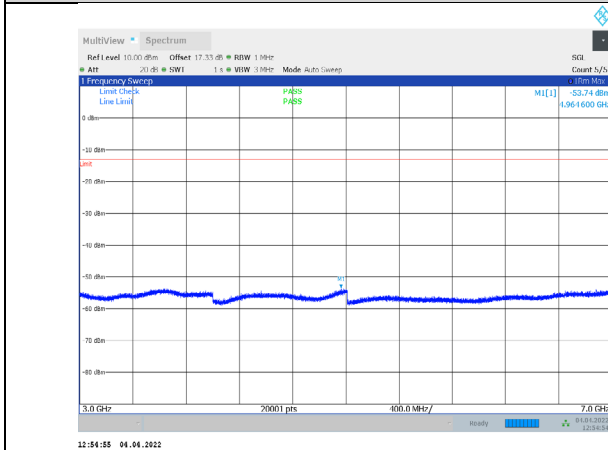
1-N71-PC3-15-20-L-1-CP-QPSK-Edge_1RB_Left-1@0 -3000-7000-Ant1--53.74--13-PASS
