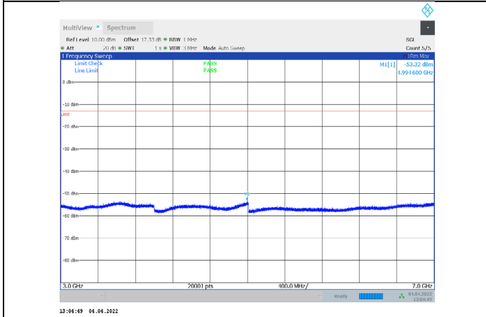
1-N71-PC3-15-20-H-3-CP-QPSK-Outet_Full-106@0-30 00-7000-Ant1--53.32--13-PASS
