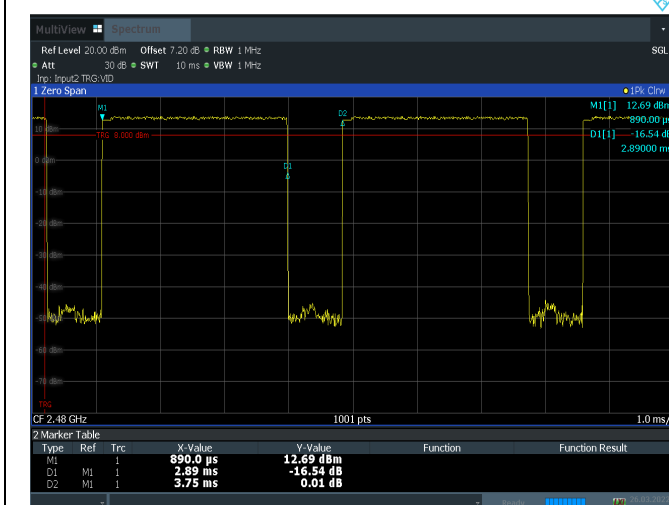
2DH5_Ant1_2480
