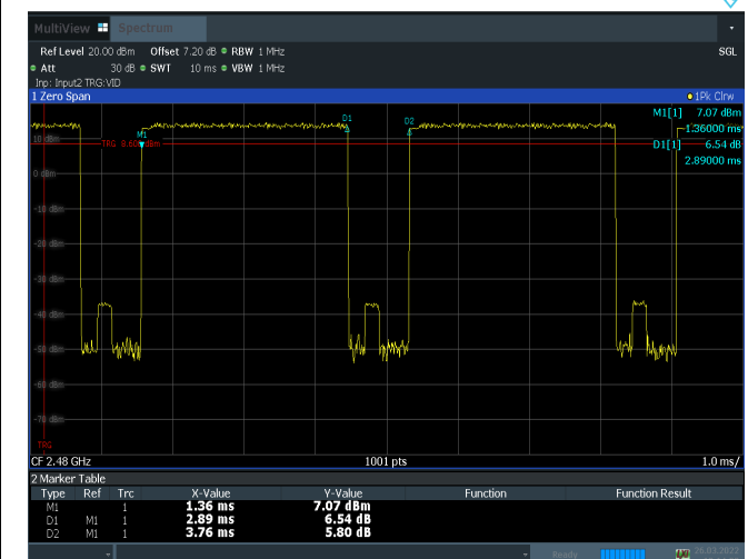
3DH5_Ant2_2480
