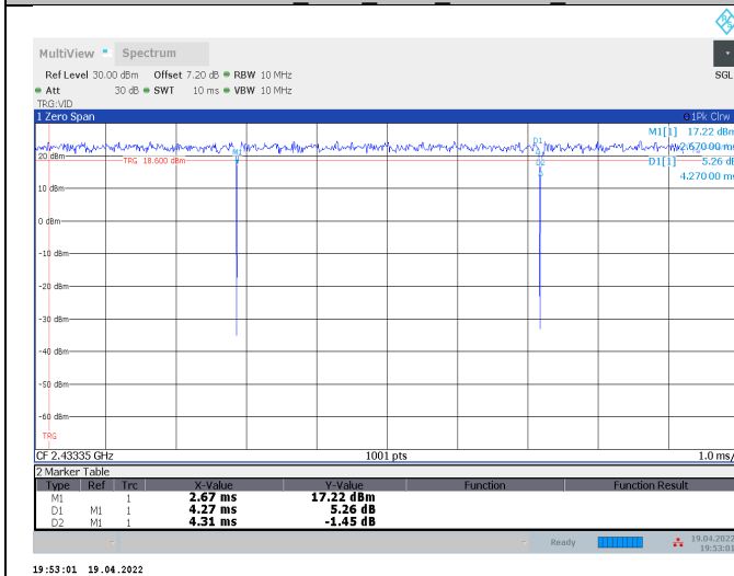
11AX20SISO_Ant2_2437_52Tone_RU37
