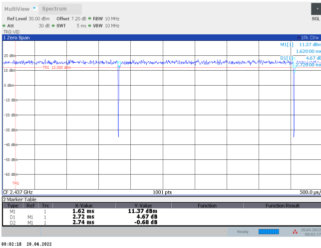
11N40MIMO_Ant1_2437
