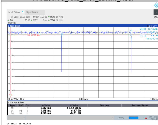
11AX20SISO_Ant2_2437_52Tone_RU37
