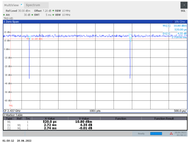
11N40MIMO_Ant2_2437
