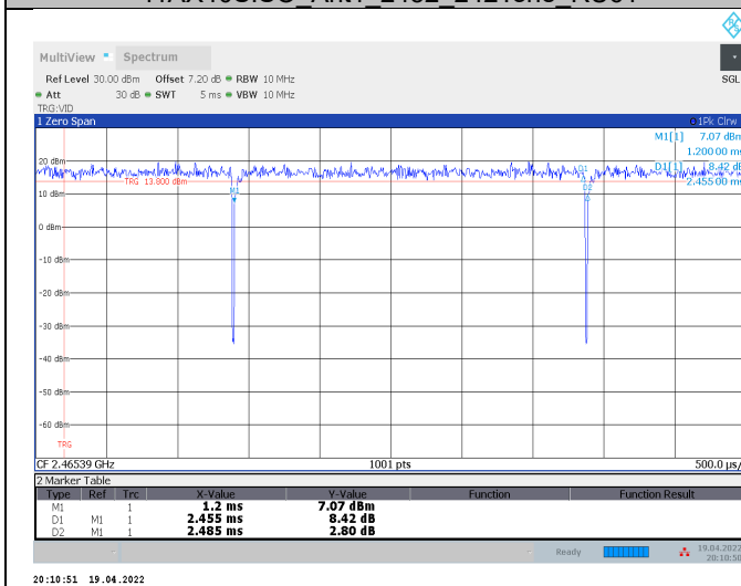
11AX40SISO_Ant1_2452_242Tone_RU61
