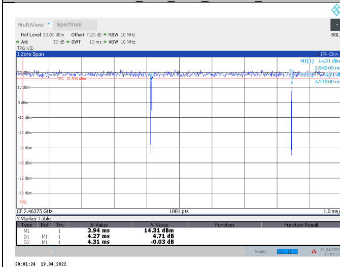
11AX20SISO_Ant2_2462_52Tone_RU37
