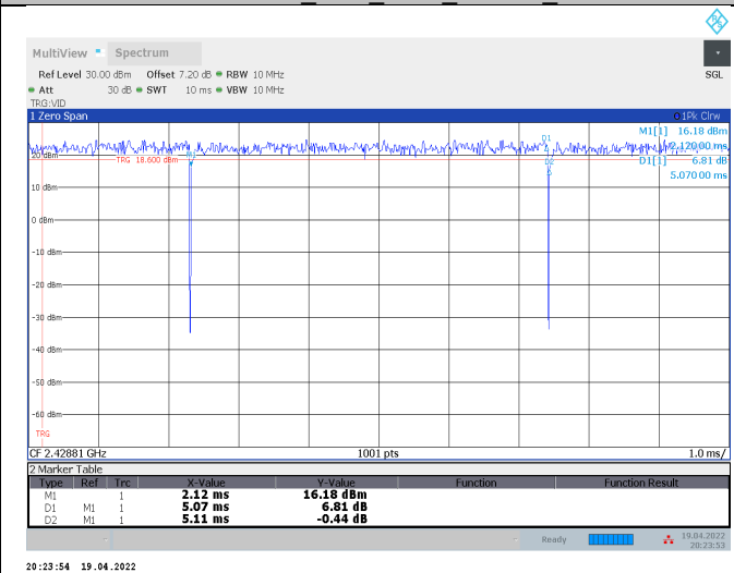
11AX20SISO_Ant2_2437_106Tone_RU53
