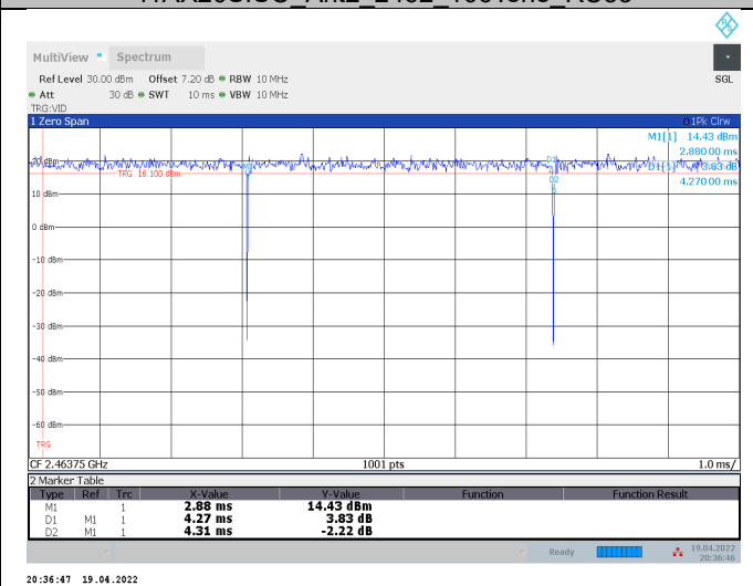
11AX20SISO_Ant2_2462_106Tone_RU53
