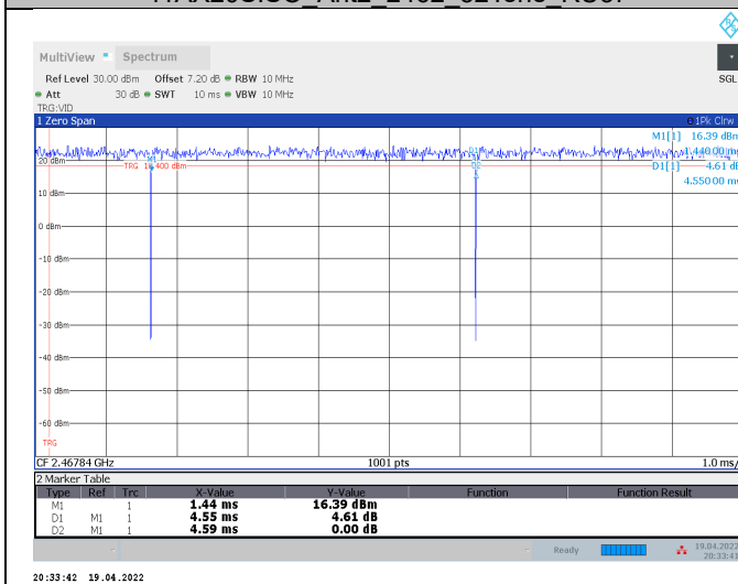
11AX20SISO_Ant2_2462_52Tone_RU37
