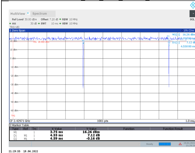
11AX20MIMO_Ant2_2437_52Tone_RU37
