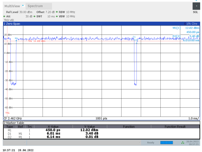
11N20MIMO_Ant2_2462
