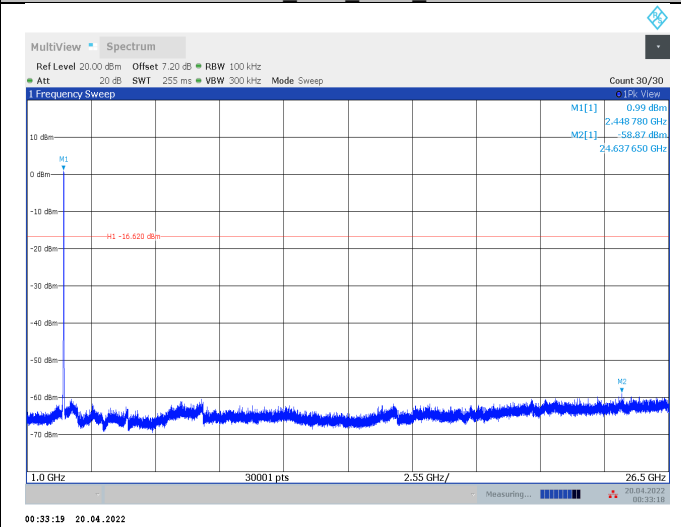
11AX20MIMO_Ant2_2452_1000~26500
