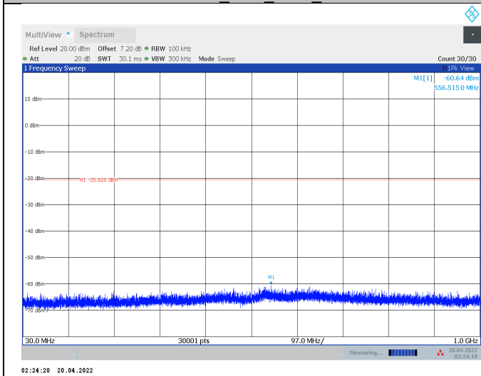
11AX40MIMO_Ant1_2452_30~1000
