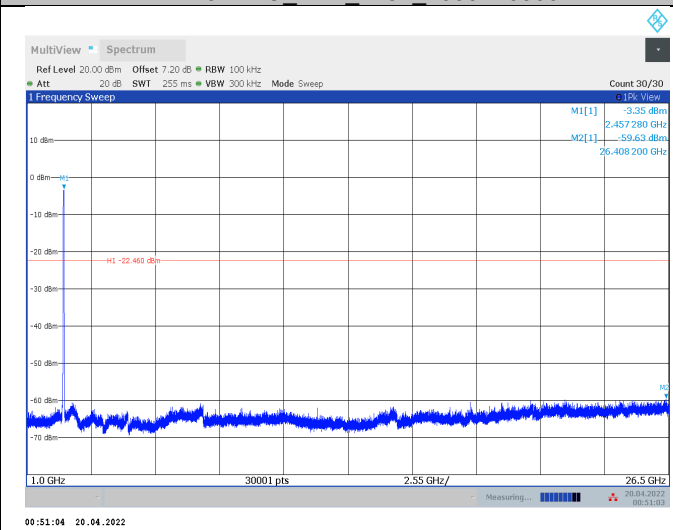
11AX40MIMO_Ant1_2452_1000~26500
