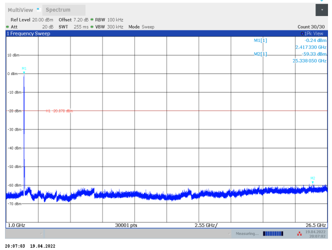
11AX40SISO_Ant2_2422_242Tone_RU61_1000~26500
