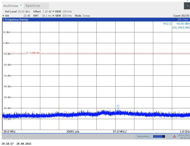
11AX20SISO_Ant2_2412_52Tone_RU37_30~1000
