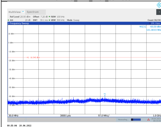
11AX20MIMO_Ant1_2457_30~1000
