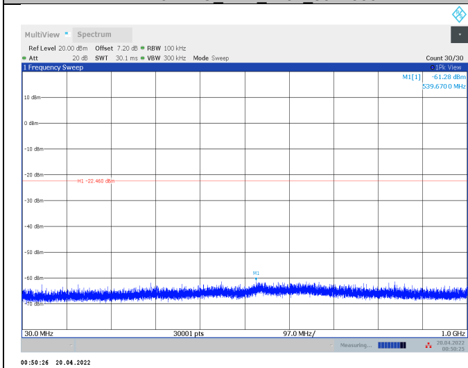
11AX40MIMO_Ant1_2452_30~1000
