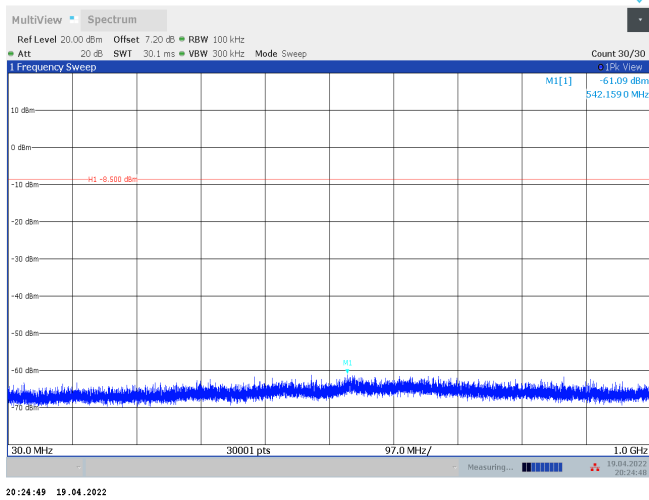
11AX20SISO_Ant2_2437_52Tone_RU37_30~1000
