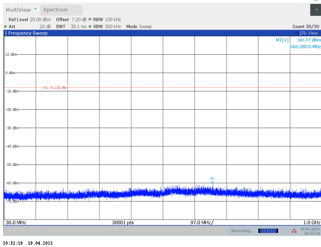
11AX20SISO_Ant2_2462_52Tone_RU37_30~1000
