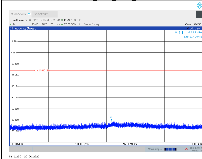
11AX20MIMO_Ant1_2462_30~1000
