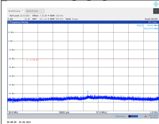
11AX40MIMO_Ant2_2447_30~1000
