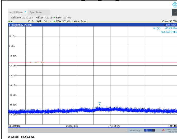
11AX20MIMO_Ant2_2452_30~1000
