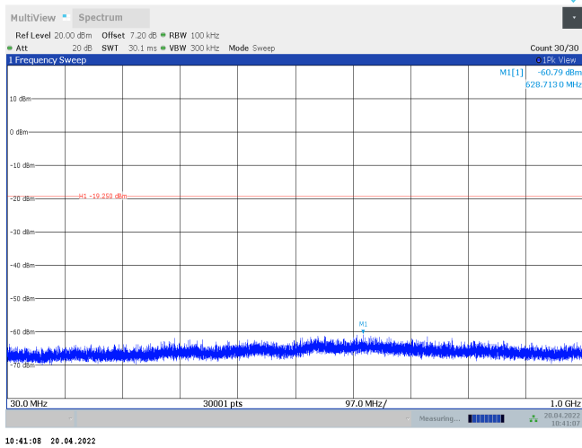
11N20MIMO_Ant1_2422_30~1000
