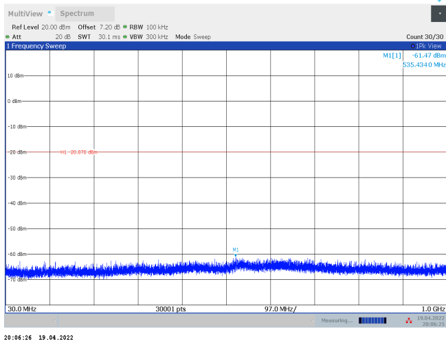
11AX40SISO_Ant2_2422_242Tone_RU61_30~1000
