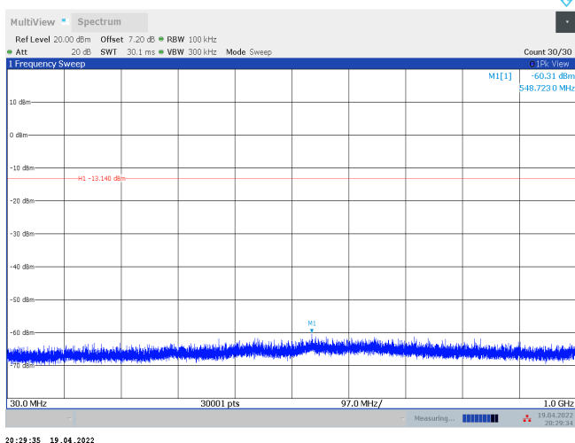
11AX20SISO_Ant2_2437_106Tone_RU53_30~1000
