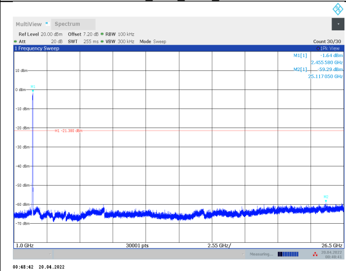
11AX40MIMO_Ant2_2447_1000~26500
