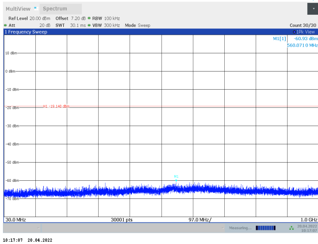
11N20MIMO_Ant2_2417_30~1000
