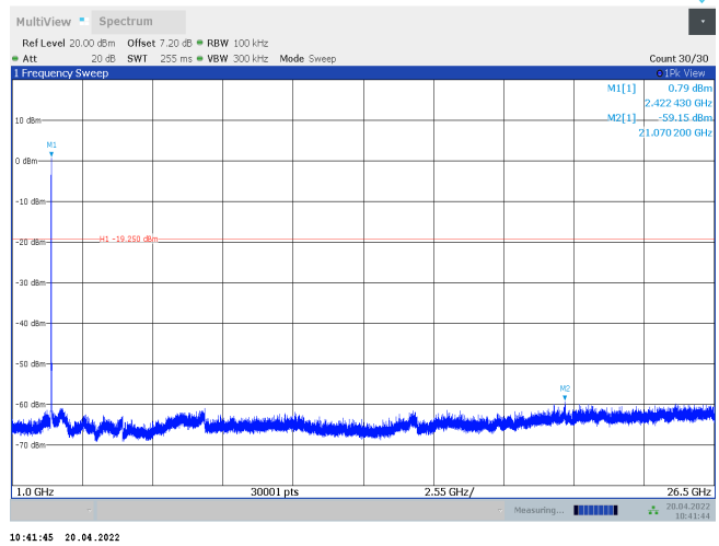
11N20MIMO_Ant1_2422_1000~26500
