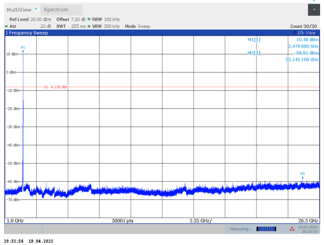
11AX20SISO_Ant2_2462_52Tone_RU37_1000~26500
