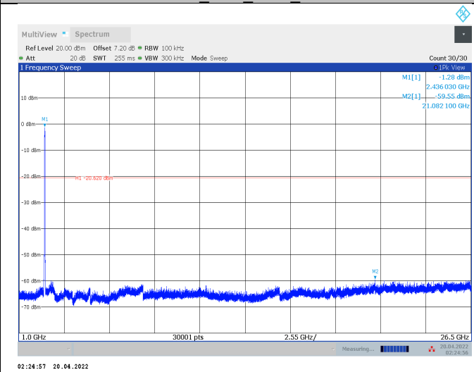
11AX40MIMO_Ant1_2452_1000~26500
