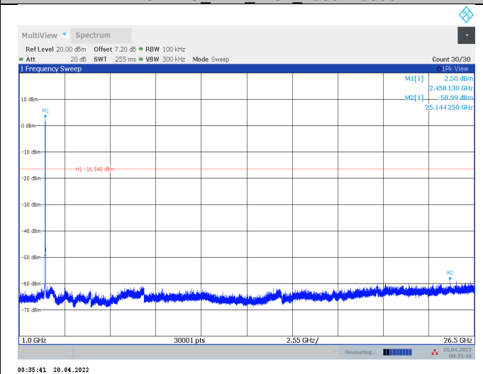
11AX20MIMO_Ant1_2457_1000~26500
