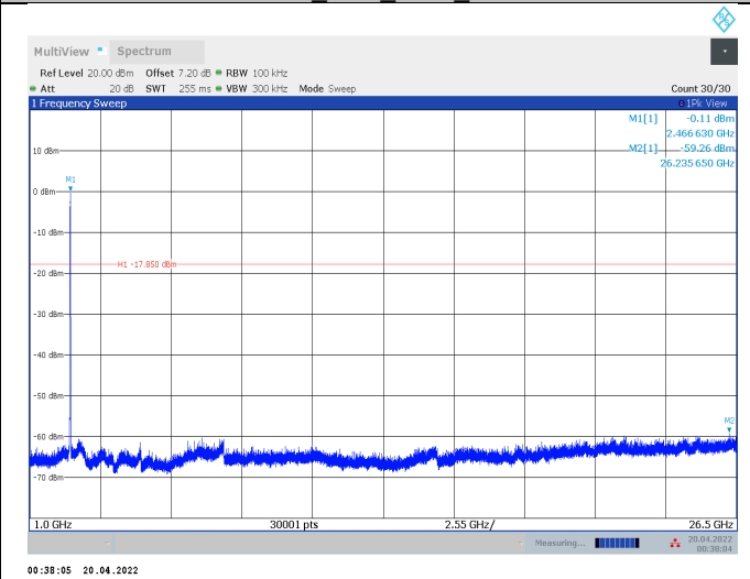
11AX20MIMO_Ant2_2462_1000~26500
