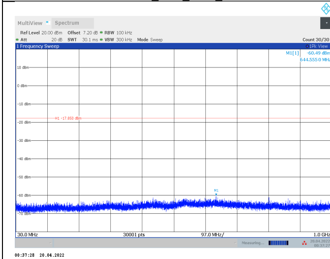
11AX20MIMO_Ant2_2462_30~1000
