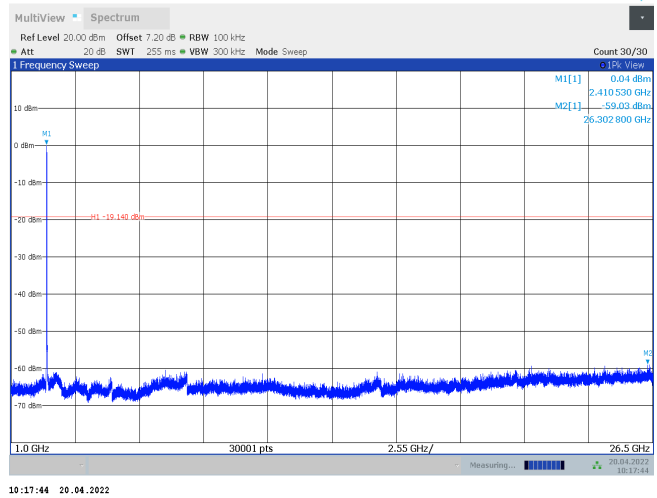
11N20MIMO_Ant2_2417_1000~26500
