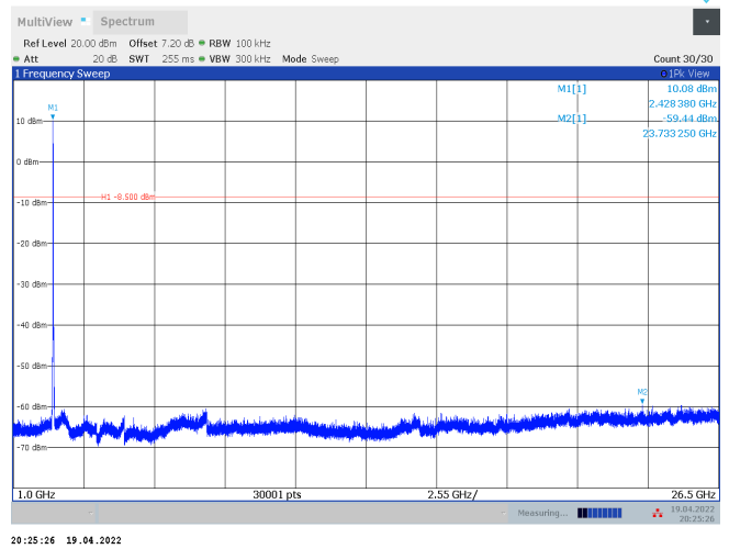
11AX20SISO_Ant2_2437_52Tone_RU37_1000~26500
