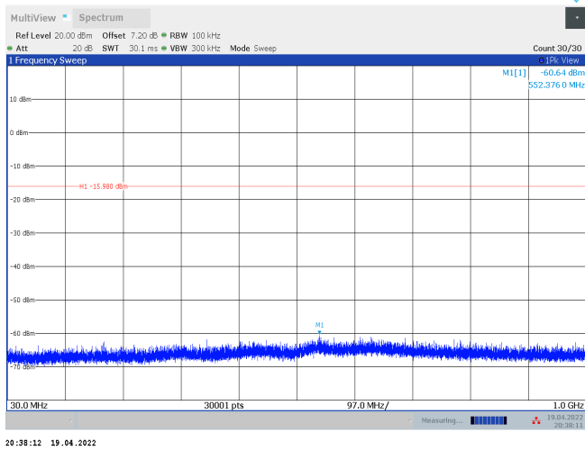
11AX20SISO_Ant2_2462_106Tone_RU53_30~1000
