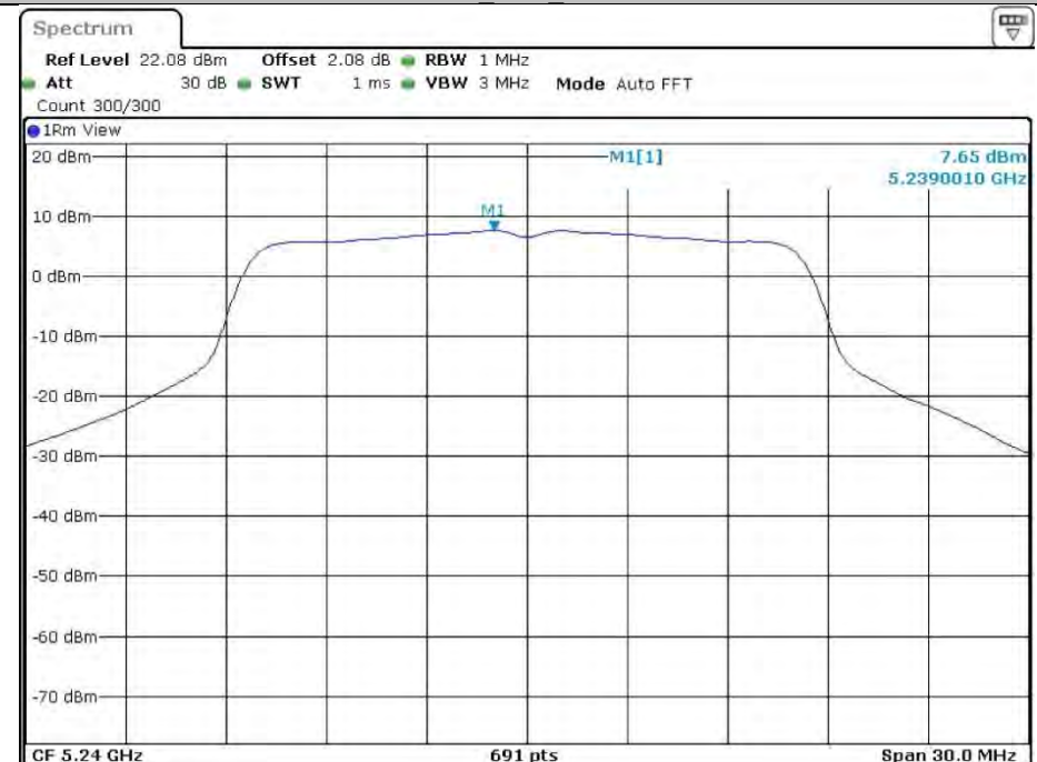
11A Ant1 5240
