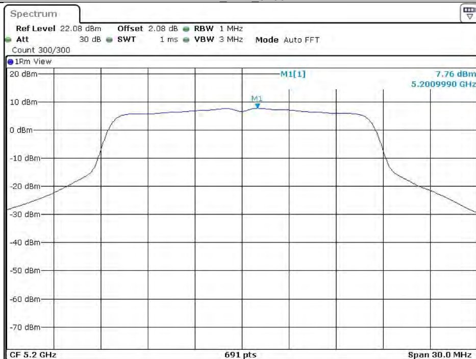
11A Ant1 5200
