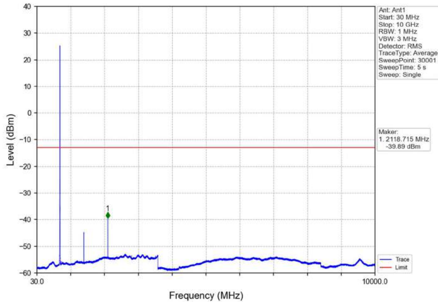
Band12_3MHz_QPSK_MCH_707.5MHz_RB_1_0_NTNV
