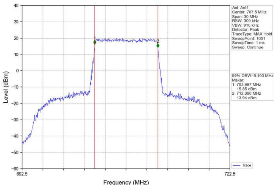
Band12_10MHz_QPSK_MCH_707.5MHz_RB_50_0_NTNV
