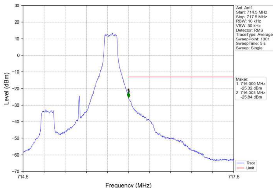
Band12_ 1.4MHz_ 16QAM_ HCH_ 715.3MHz_ RB_ 1_ 5_ NTVN
