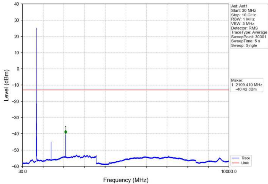
Band12_10MHz_QPSK_MCH_707.5MHz_RB_1_0_NTNV
