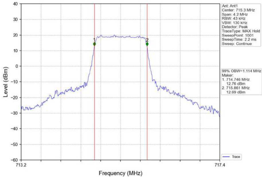
Band12_ 1.4MHz_ 16QAM_ HCH_ 715.3MHz_ RB_ 6_ 0_ NTVN
