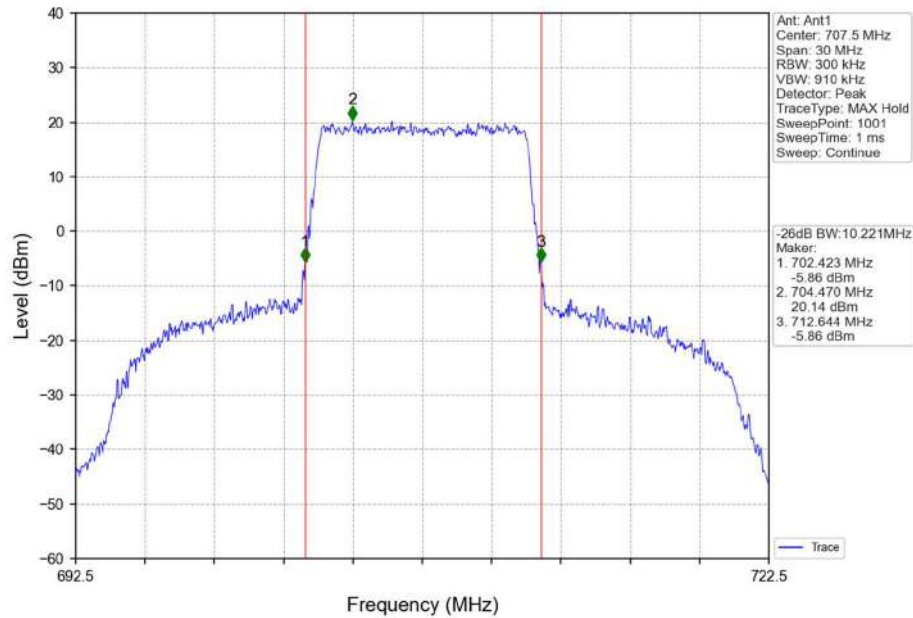
Band12_10MHz_QPSK_MCH_707.5MHz_RB_50_0_NTNV
