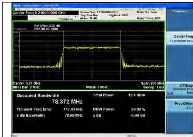
Test Mode:802.11be EHT80 5210MHz Chain0
