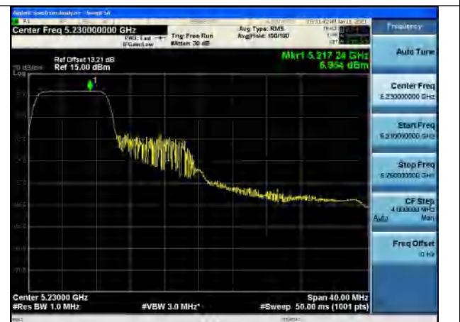
Test Mode:802.11be EHT40 5230MHz Chain1
