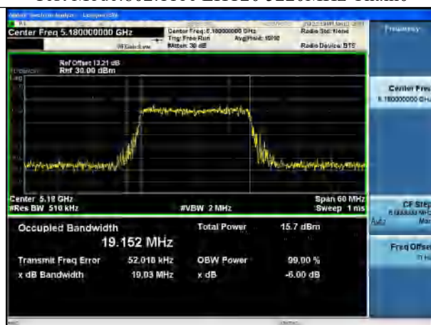
Test Mode:802.11be EHT20 5180MHz Chain1
