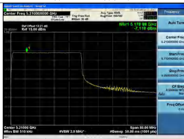
Test Mode:802.11be EHT80 5210MHz Chain1
