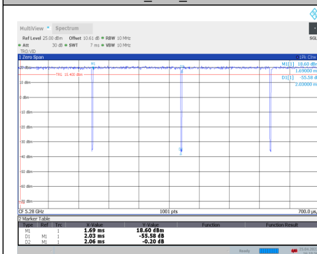
11A_Ant1_5280
