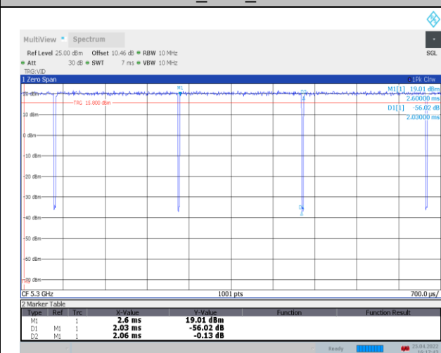
11A_Ant1_5300
