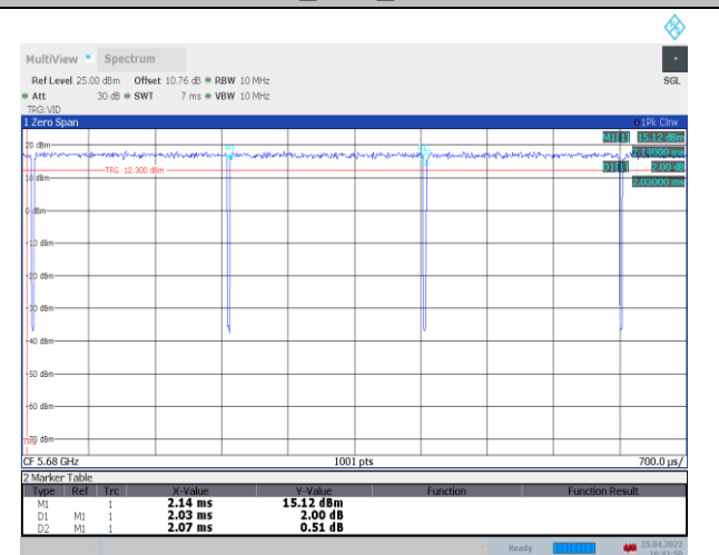
11A_Ant1_5680
