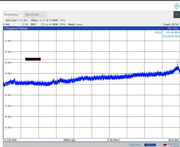
11N40ISO_Ant1_5670_5735~40000
