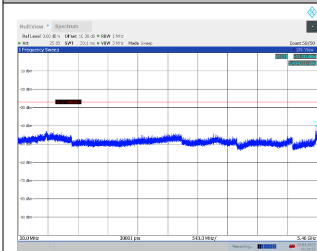
11A_Ant1_5520_30~5460
