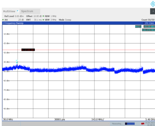
11A_Ant1_5680_30~5460
