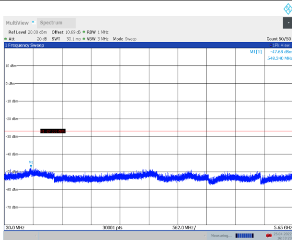
11A_Ant1_5825_30~5650
