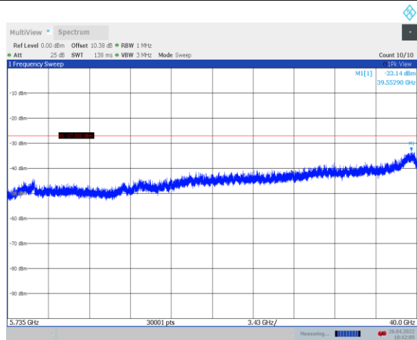
11N40ISO_Ant1_5630_5735~40000
