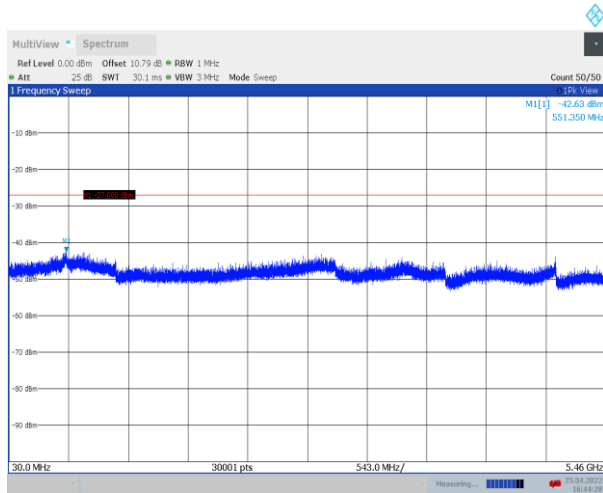
11A_Ant1_5720_30~5460
