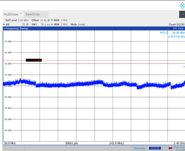
11N20SISO_Ant1_5580_30~5460
