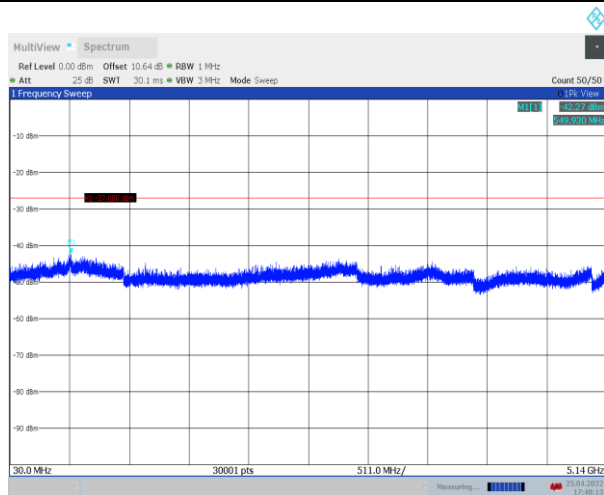
11N40SISO_Ant1_5230_30~5140
