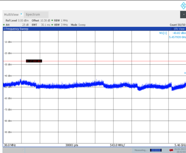
11N40ISO_Ant1_5630_30~5460
