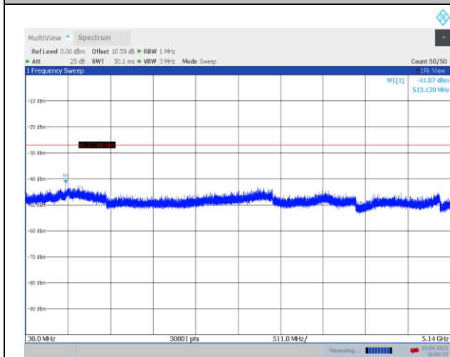
11A_Ant1_5280_30~5140
