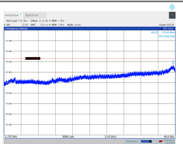
11A_Ant1_5520_5735~40000
