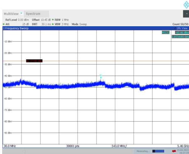
11A_Ant1_5660_30~5460
