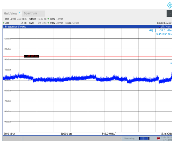
11N20SISO_Ant1_5520_30~5460
