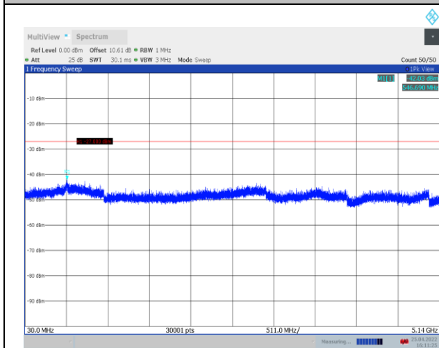
11A_Ant1_5300_30~5140
