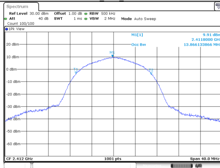
11B Ant0 2412
