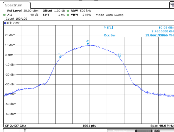
11B Ant0 2437
