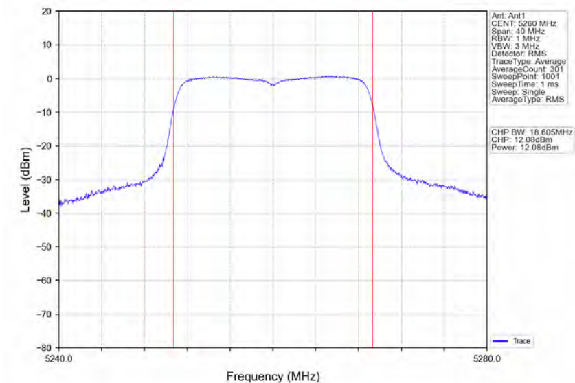
802.11n(HT20)_LCH_5260MHz_Ant1_NTNV
