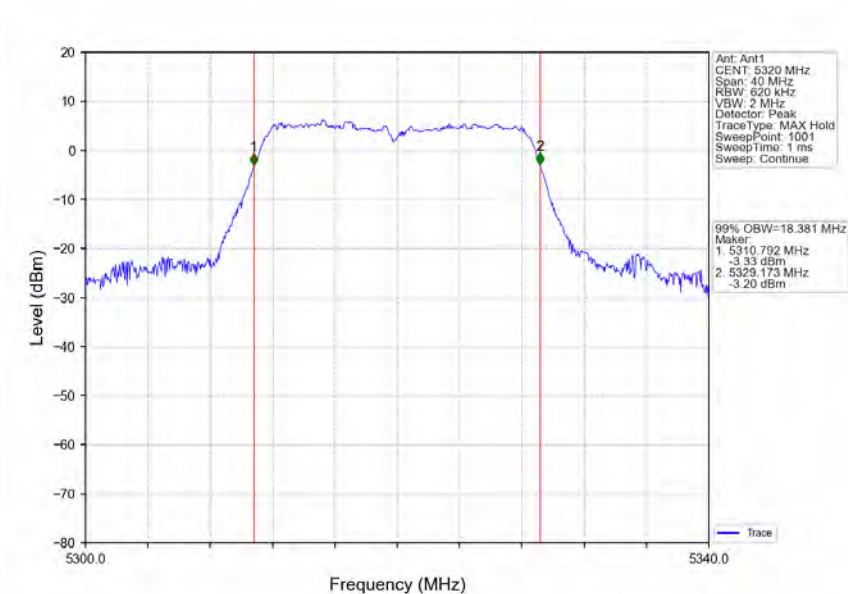
802.11n(HT20)_HCH_5320MHz_Ant1_NTNV
