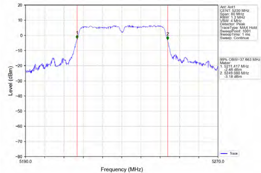
802.11ac(VHT40)_HCH_5230MHz_Ant1_NTNV
