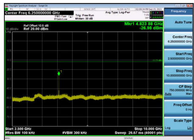
,Plot 4,2500MHz~10000MHz-802.11b
