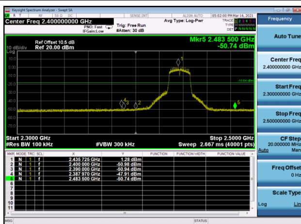
,Plot 2,Band Edge-802.11n(HT20) ,2437MHz
