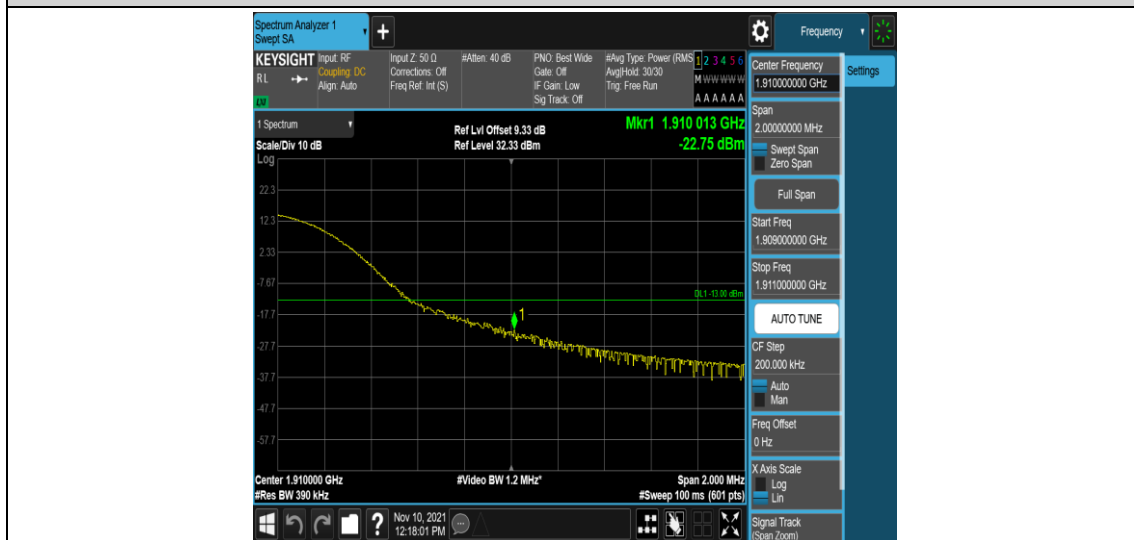
Band2-20MHz-QPSK-19100-1RB#99
