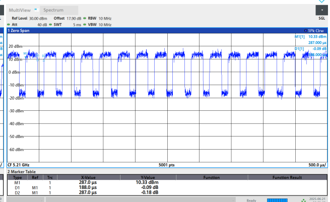
802.11ac(VHT80)
