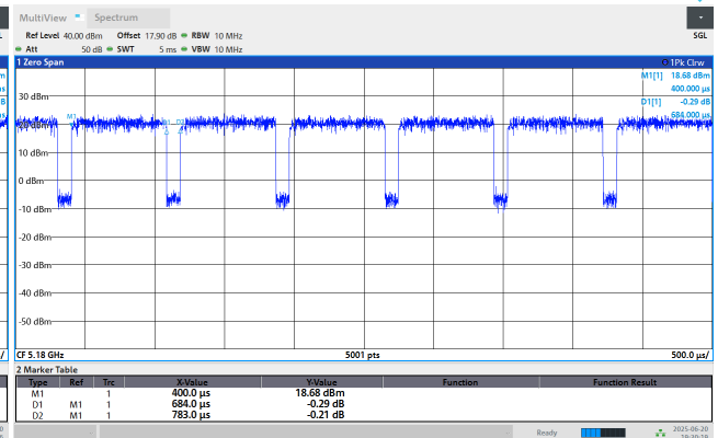
802.11ac(VHT20)
