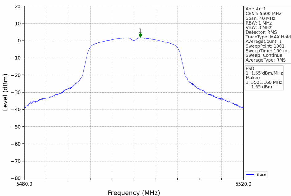
802.11n(HT20)_LCH_5500MHz_Ant1_NTNV
