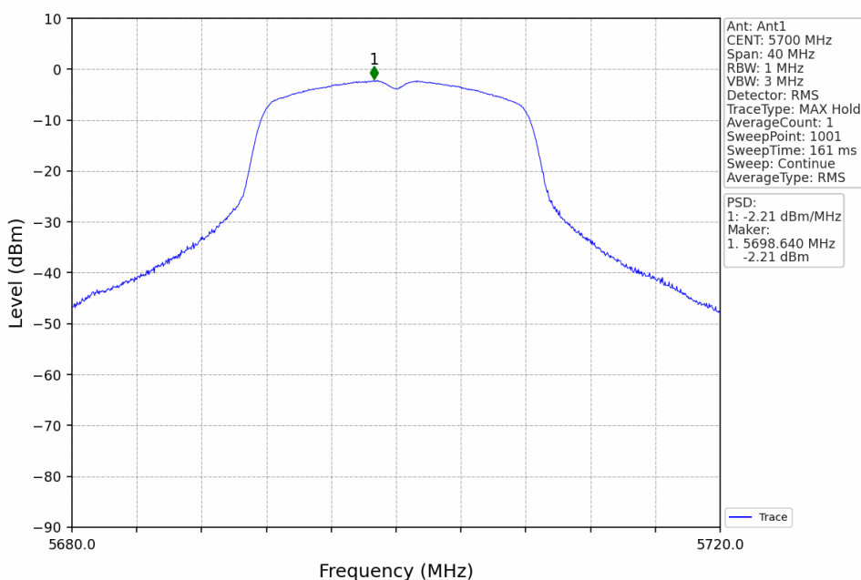
802.11n(HT20)_HCH_5700MHz_Ant1_NTNV
