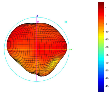
Total_3D_E2_5.85GHz
