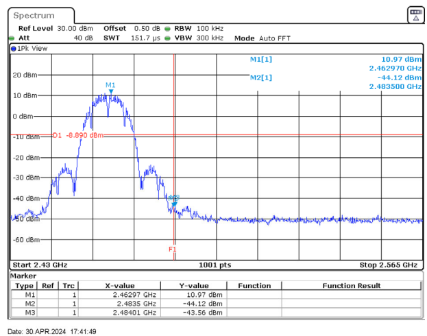
802.11g / 2462 MHz
