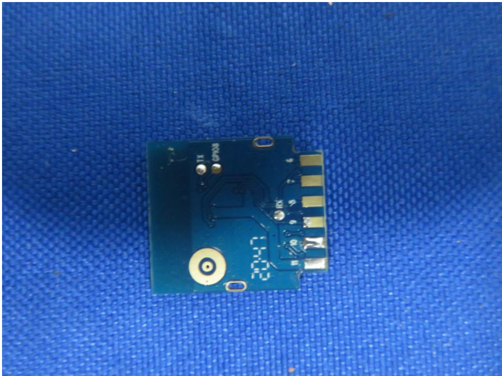
BT&WIFI ANT
