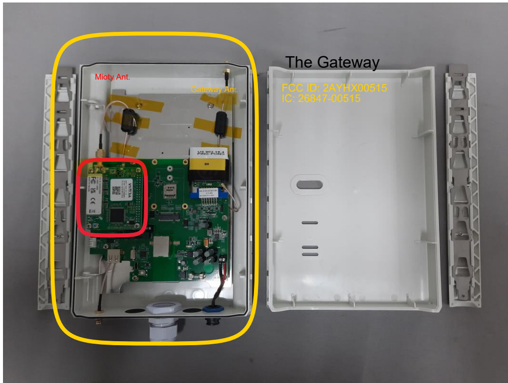
Mioty module
