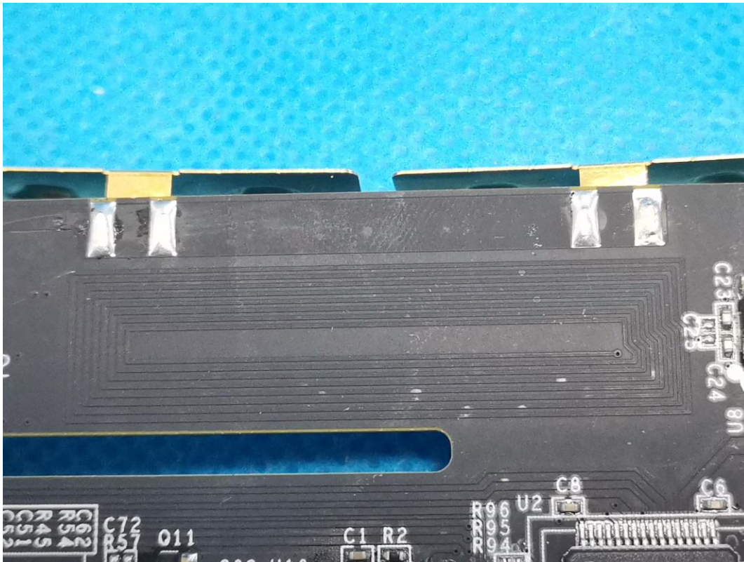
NFC Antenna
