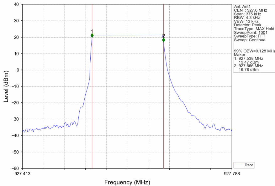
LORA_HCH_927.6MHz_Ant1_NTNV
