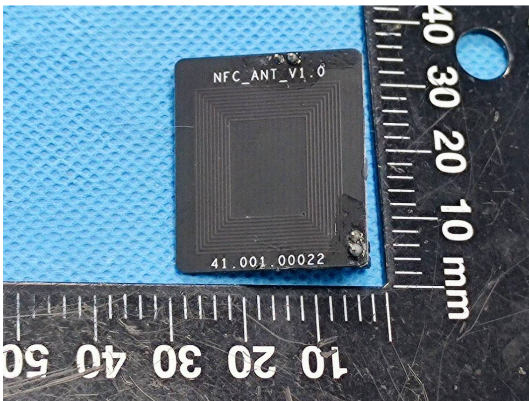
NFC Antenna
