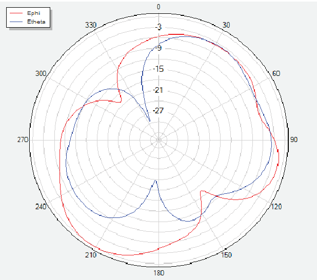
Theta=90 freq=2500MHz
