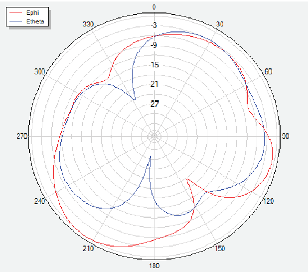
Theta=90 freq=2400MHz
