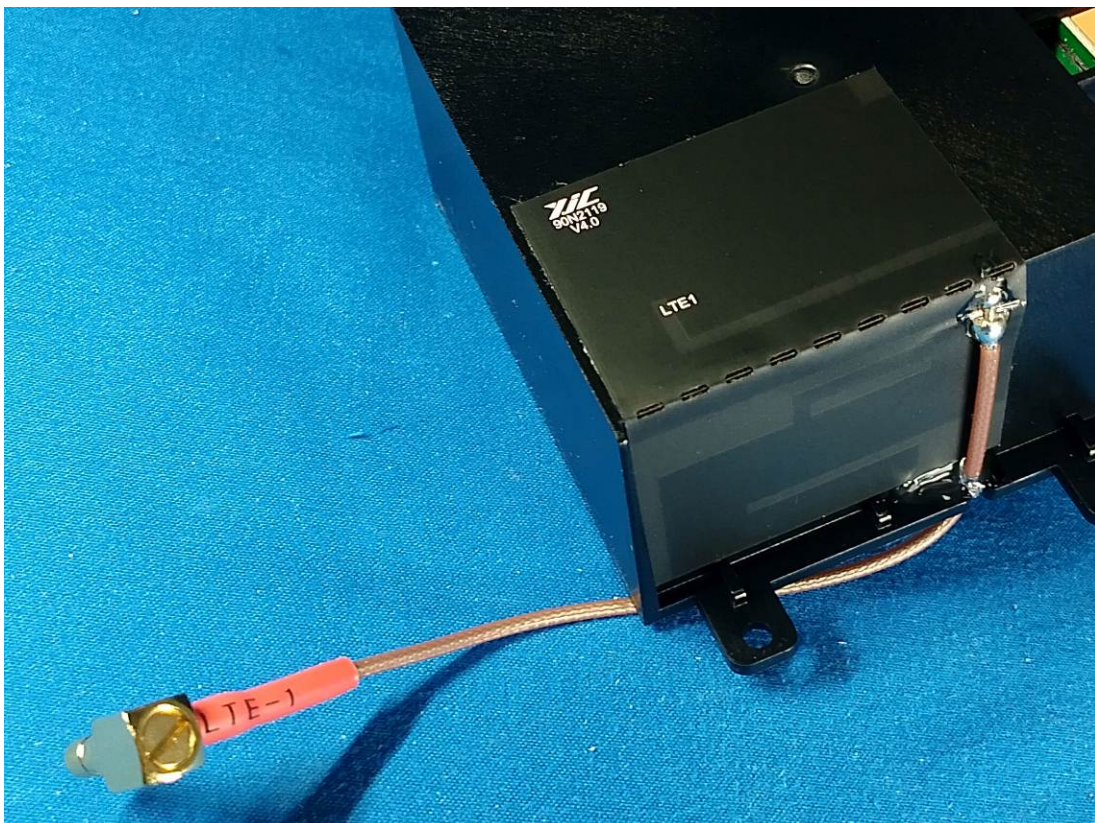
WWAN Antenna(LTE 1)
