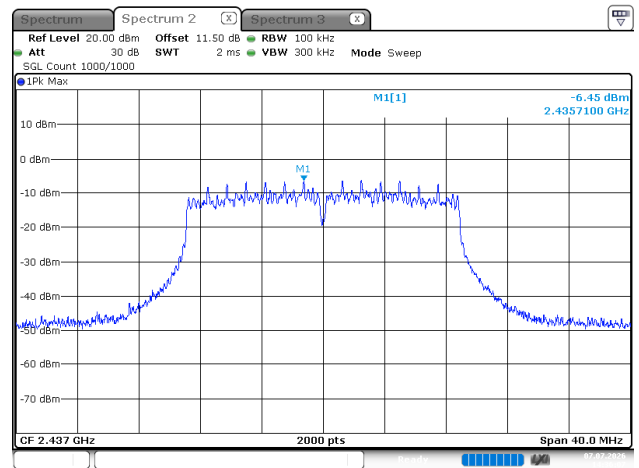
802.11n20_2437MHz_Chain 1
