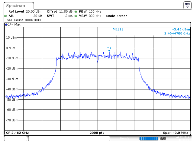
802.11n20_2462MHz_Chain 1
